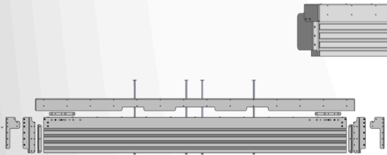
60 x 290 mm 4 Kalkar Montajlı
